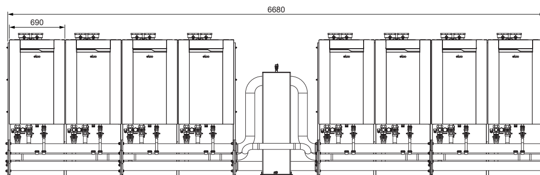
THISION L PLUS — монтаж на раме в ряд 8 котлов
